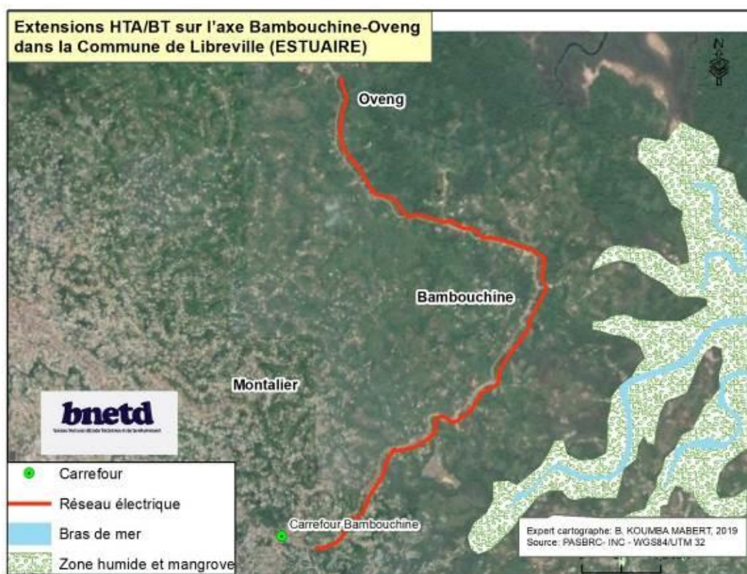
Figure 4- Axes pour les travaux d'extension et de renforcement des lignes HTA/BT à Libreville
